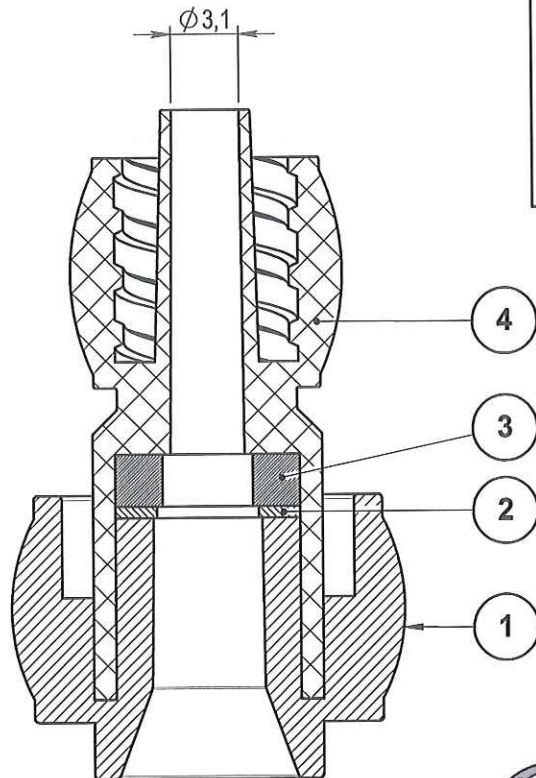
COUPE A-A
