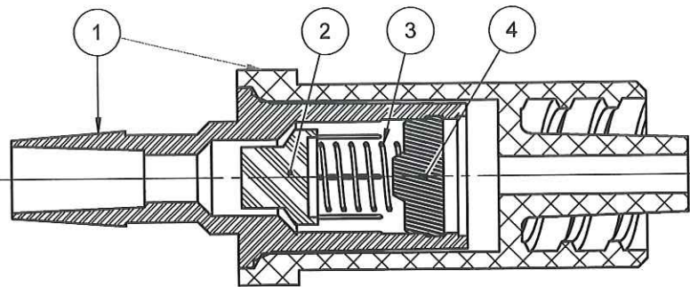
COUPE A-A
