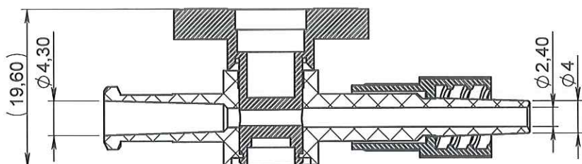
COUPE A-A
