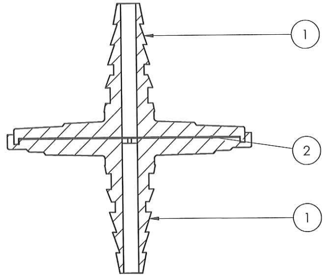
COUPE A-A
