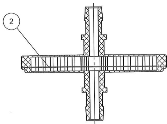
COUPE A-A
