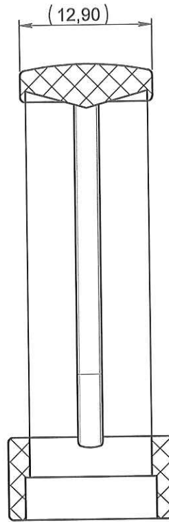
COUPE A-A
