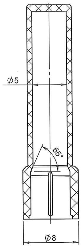
COUPE A-A
