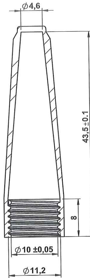
COUPE A-A
