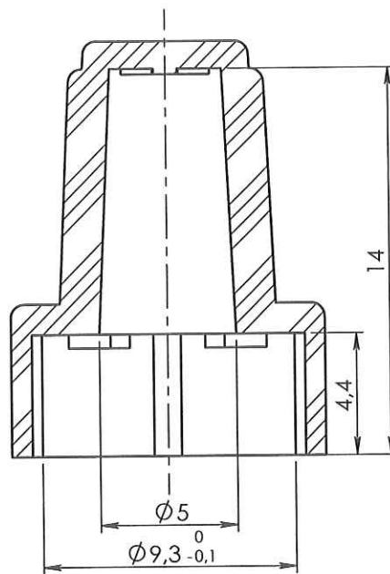
COUPE A-A ECHELLE 4 : 1
