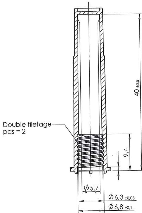
COUPE A-A
