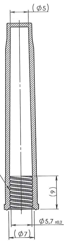
COUPE A-A
