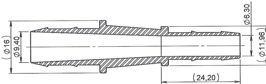
COUPE A-A
