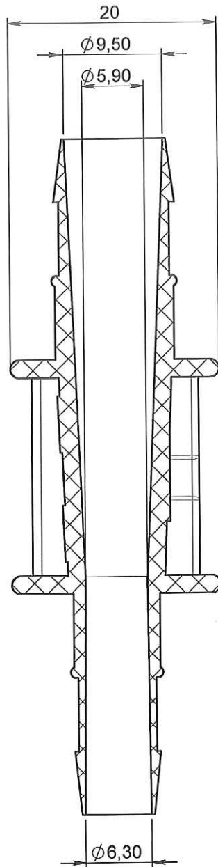
COUPE A-A
