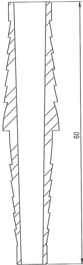
COUPE A-A
