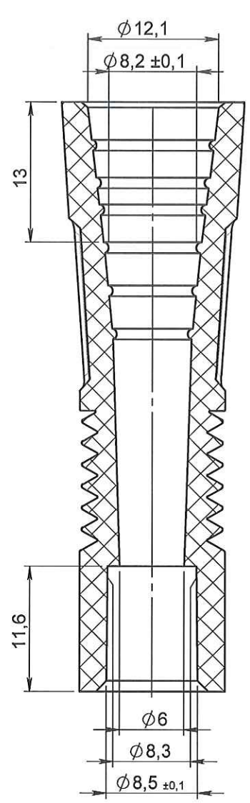
COUPE A-A
