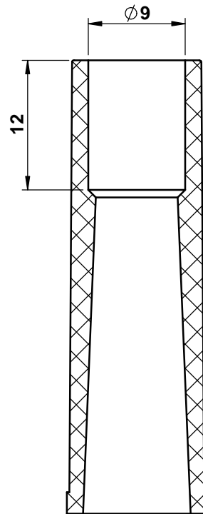
COUPE A-A
