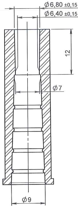
COUPE A-A
