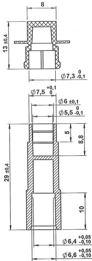
COUPE A-A VUE ECLATE
