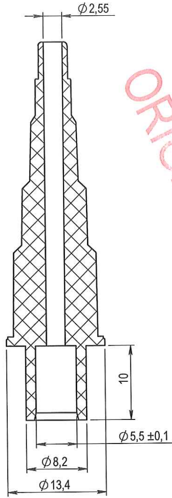
COUPE A-A
