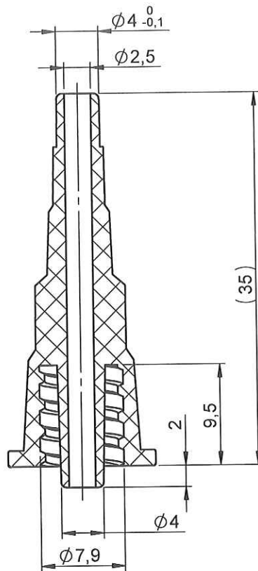
COUPE A-A
