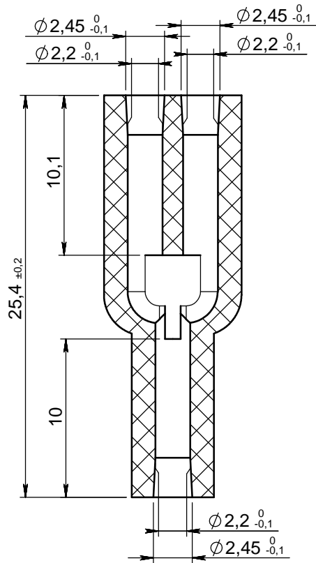
COUPE A-A
