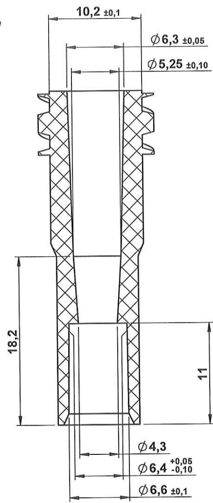
COUPE A-A ECHELLE 5 : 2
