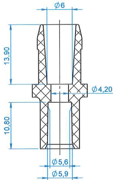
COUPE A-A
