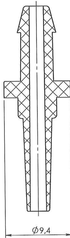
COUPE A-A
