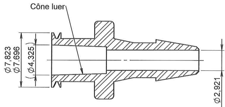
COUPE A-A
