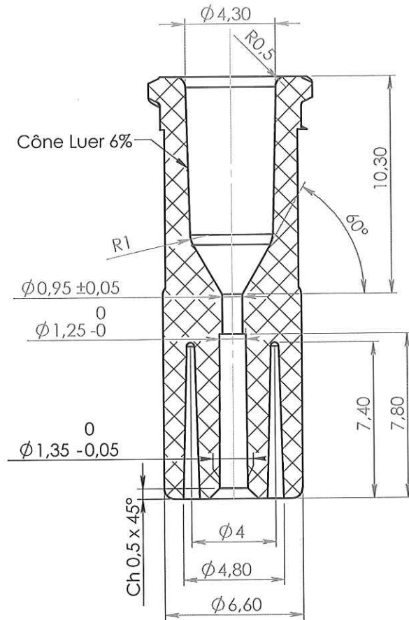
COUPE B-B Echelle 4 : 1
