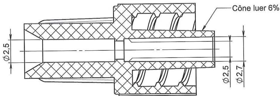
COUPE A-A
