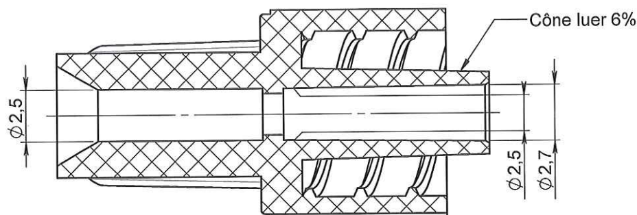
COUPE A-A
