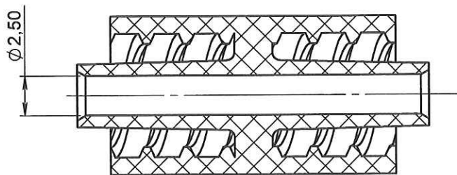
COUPE A-A
